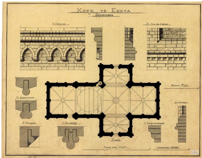
Plattegrond en details, technische tekening van C.H. Peters, 1870-1871. Collectie Groninger Archieven, verzameling Peters
